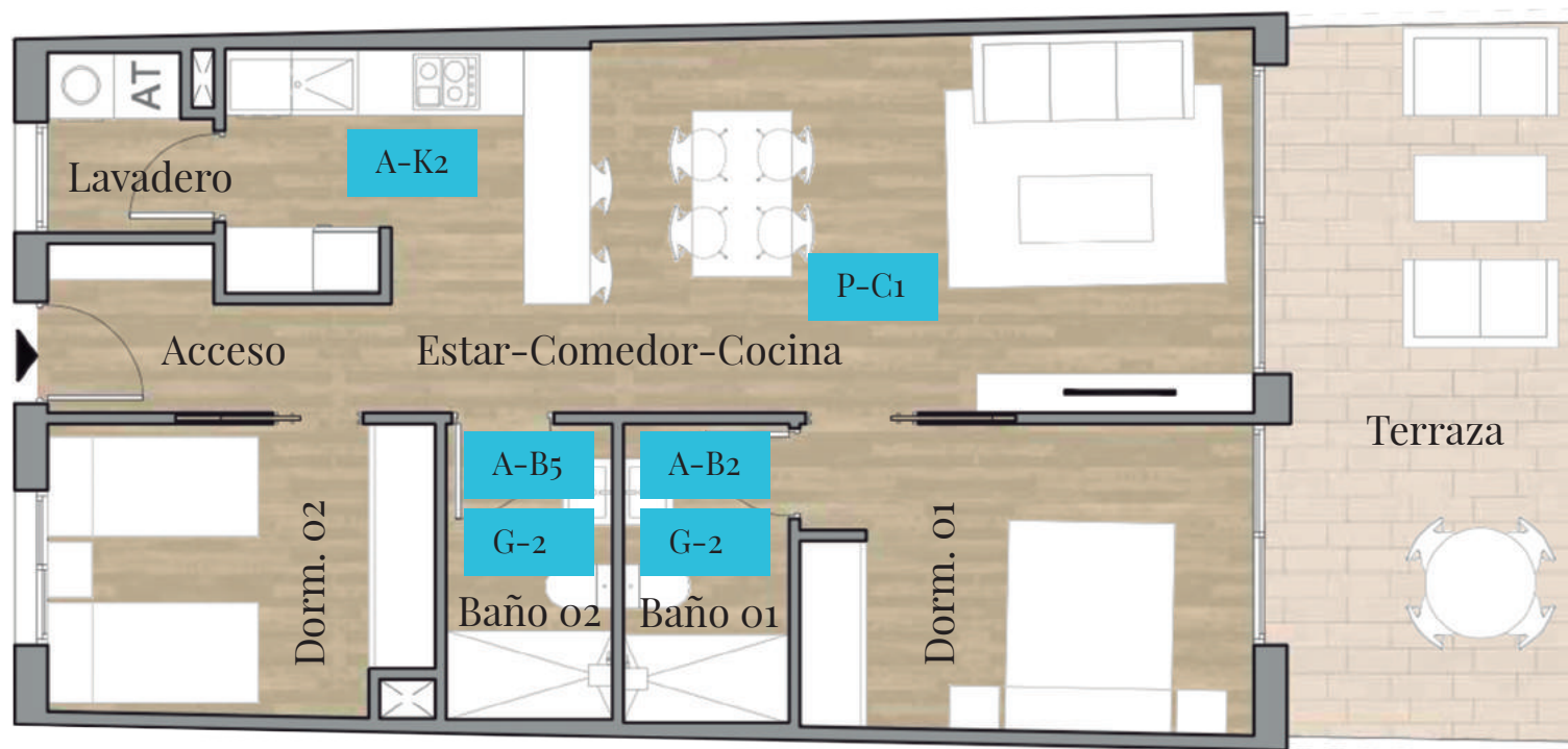
Tipo A (2 dorm.)
